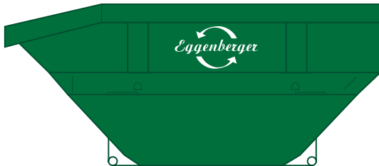
7,0 m 3 Mulde: 405 cm lang, 171 cm breit, 160 cm hoch Material: Alteisen, Metalle, Bauschutt, Papier, Holz, Sperrgut etc.
