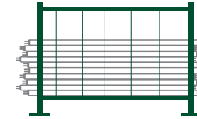
Rungenpalette: 120 cm lang, 100 cm breit, 117 cm hoch Material: FL-Röhren
