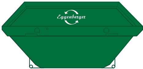
6,0 m 3 Deckelmulde: 350 cm lang, 140 cm breit, 160 cm hoch Material: Alteisen, Metalle, Bauschutt, Papier, Holz, Sperrgut etc.
