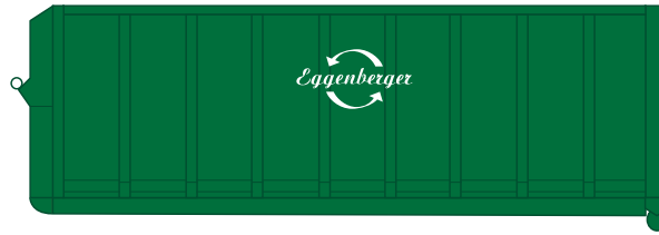
20,0 m 3 Abrollcontainer: 700 cm lang, 230 cm breit, 130 cm hoch Material: Alteisen, Bauschutt, Papier, Holz, Sperrgut, Kunststoff etc.
